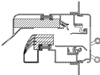
→ GlasMax 'ZR' compacte kalfplaatsing
