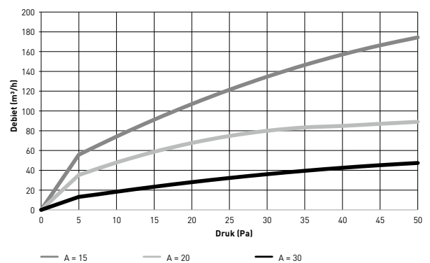
Druk / debiet curve DucoVent Basic
